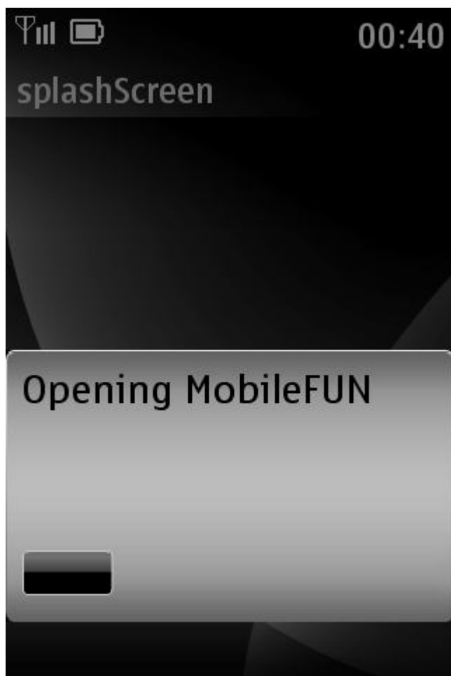
Рисунок 1: Открытие мидлета.
