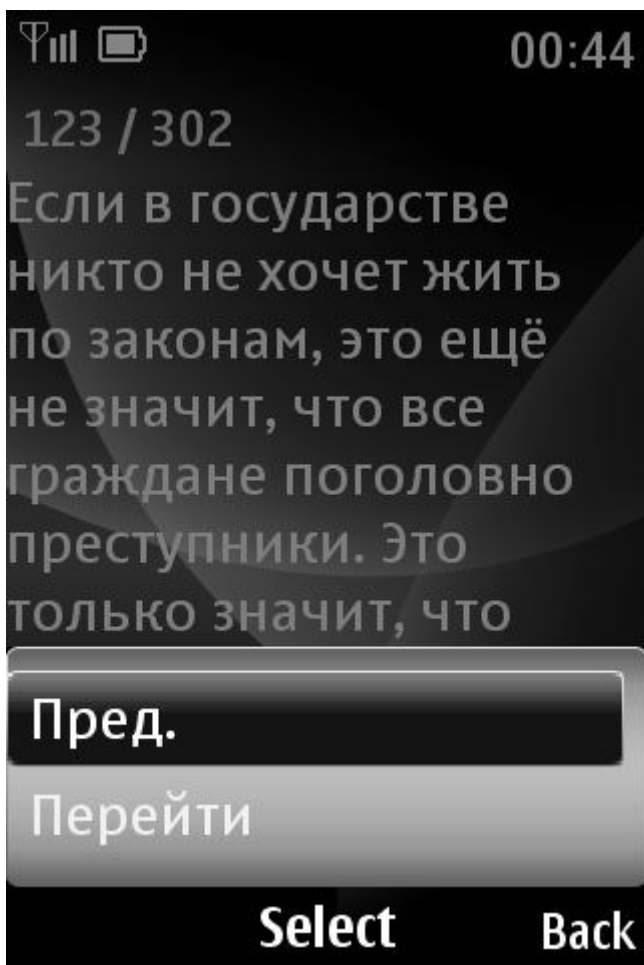
Рисунок 5 – Комманда “Пред.”
