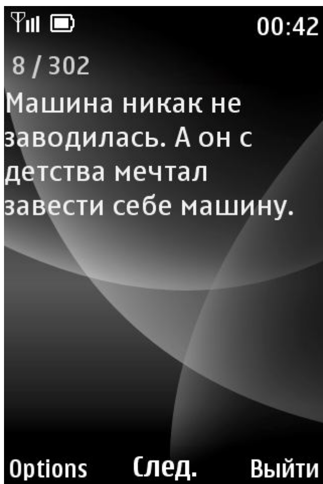
Рисунок 3 – Основное окно.
