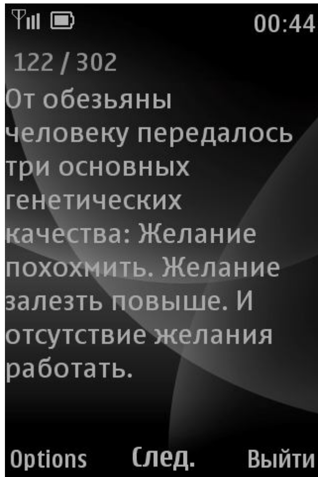
Рисунок 6 – Предыдущая фраза
