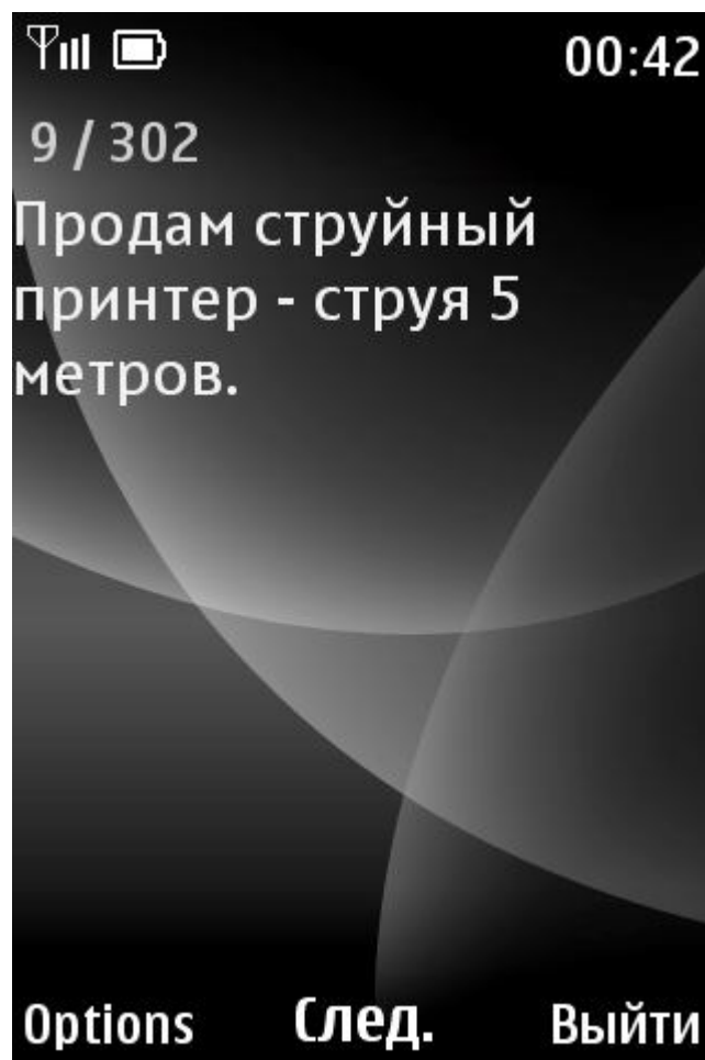
Рисунок 4 – Следующий экран.
